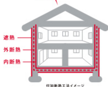
付加断熱工法イメージ
